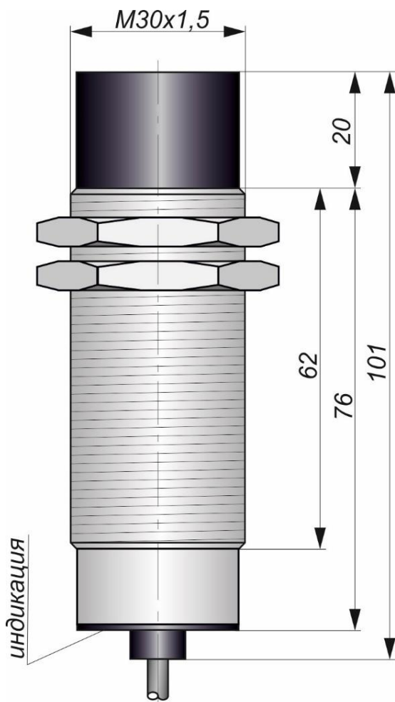
Габаритный чертеж
