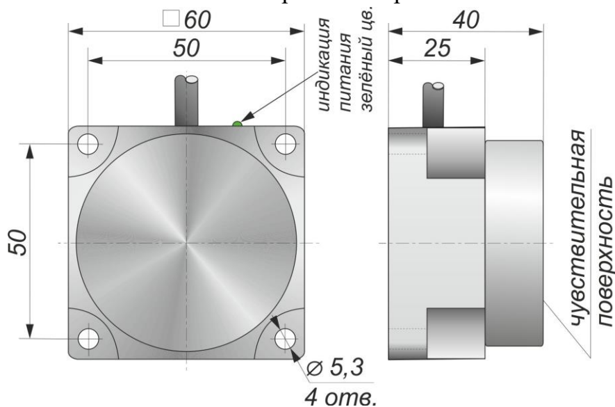
Габаритный чертеж
