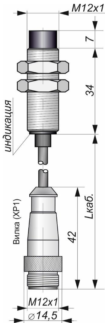
Габаритный чертеж
