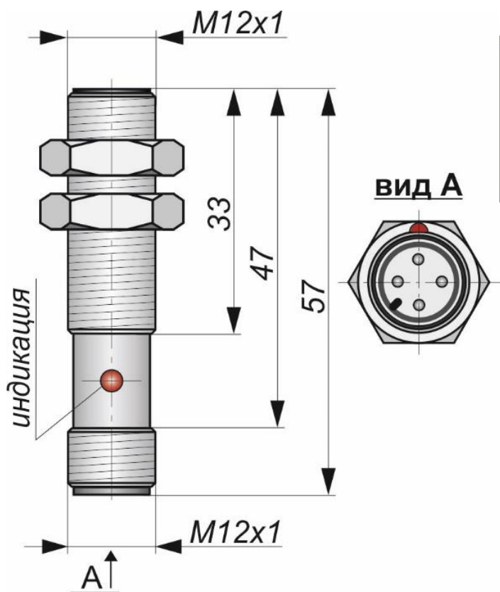
Габаритный чертеж
