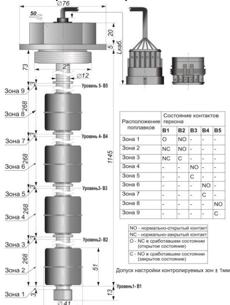
Габаритный чертёж
