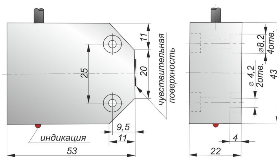
Габаритный чертеж
