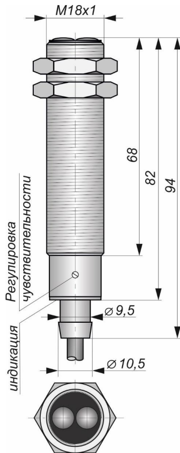
Габаритный чертеж
